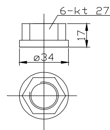
Nakrętka NK/ M20
