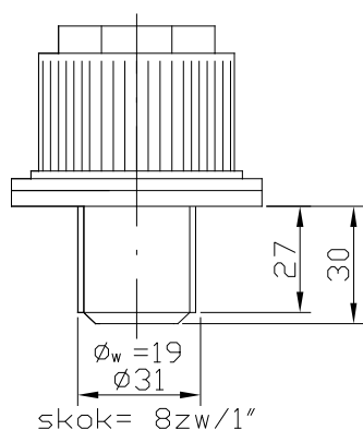
P3/30-8zw/1"
