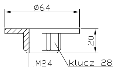
NP/M24
