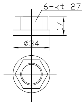
Nakrętka NK/ M20
