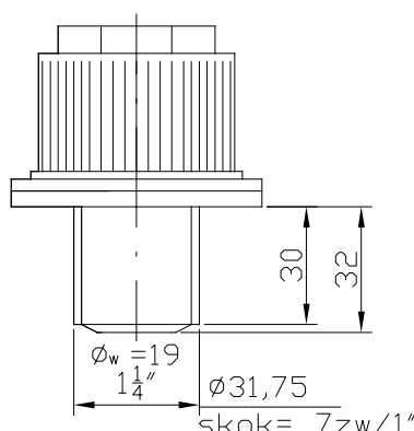
P4/30
