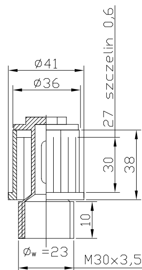
DSM30x3,5
