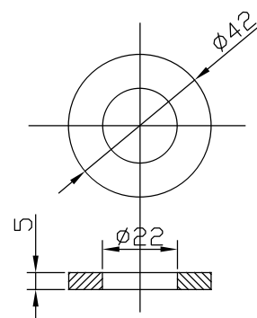
Podkładka PK-22
