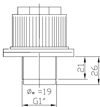
DG 1"/25
