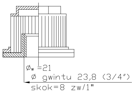
typ P5/1
