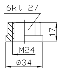
NK/M24
