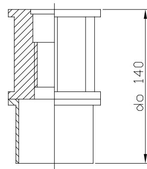
Gniazdo- nakrętka GN/M27/ X GN/M24/ X GN/W/ X
