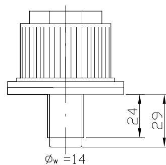
P1/20
