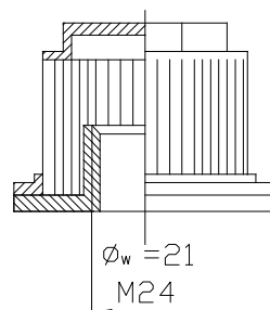
typ P5/M24
