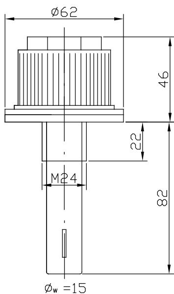
DM 24/K1
