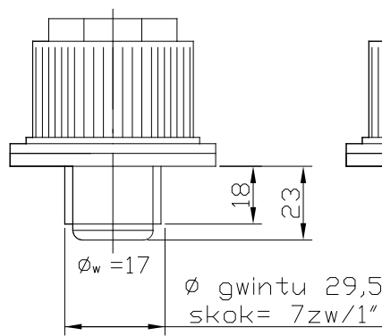
P3/20
