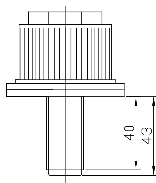
DM 20/40
