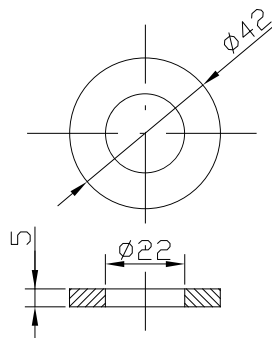
Podkładka PK-22
