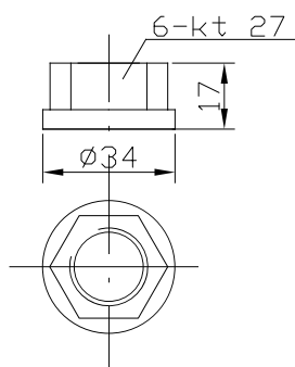
Nakrętka NK/ P1
